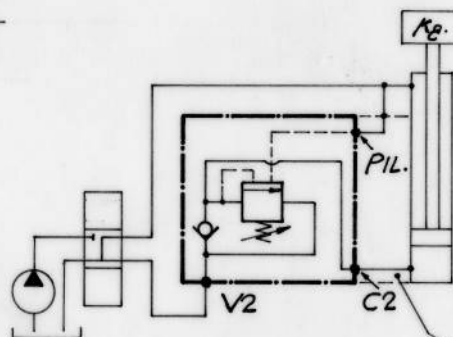
SCHEMA FUNZIONALE
