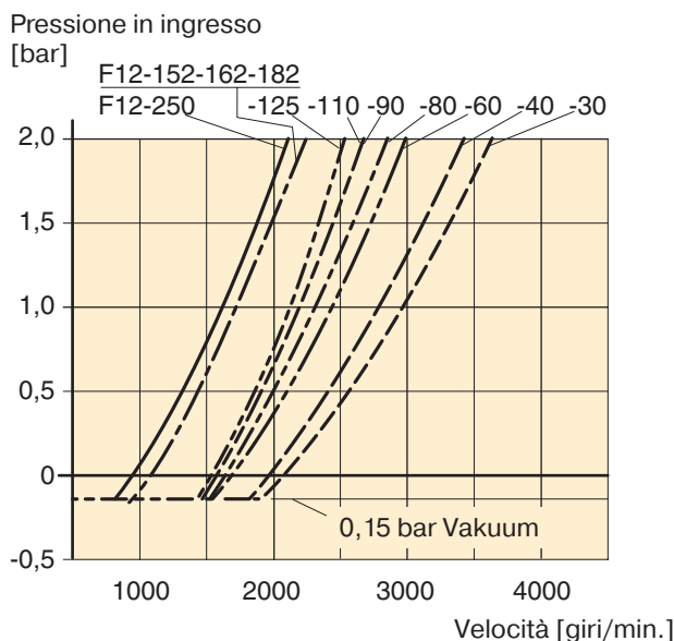
Diagramma 3. Pressione in ingresso min richiesta motore (F12-M).
