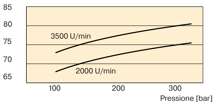
Rumorosità [dB(A)]
