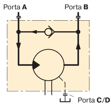
Schema del motore per ventole con valvola anticavitazione
