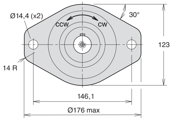
Flangia di montaggio tipo S SAE 'B' (SAE J744c)
