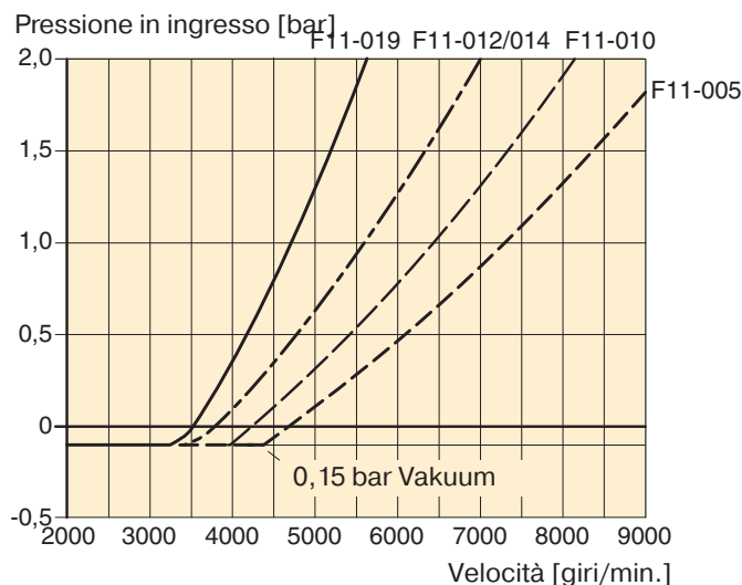
Diagramma 2. Pressione in ingresso min richiesta
