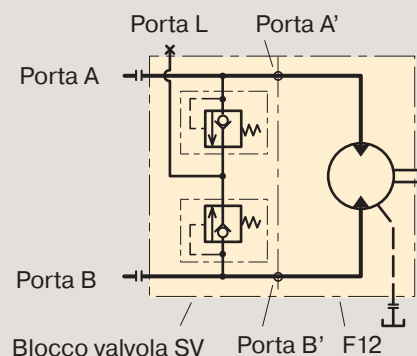
Schema idraulico
