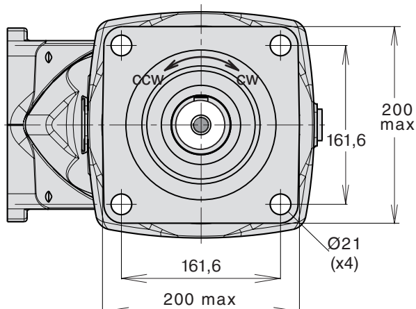
Flangia di montaggio tipo S SAE 'D' (SAE J744c)
