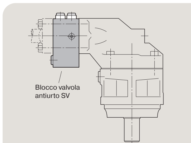
Blocco valvola SV installato su un motore F12.
