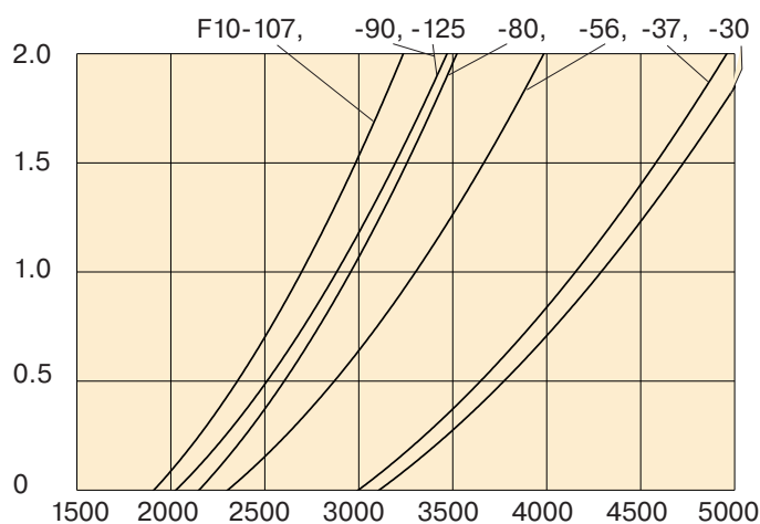
Diagramma 1 Pressione in ingresso min richiesta (F10-L o R)
