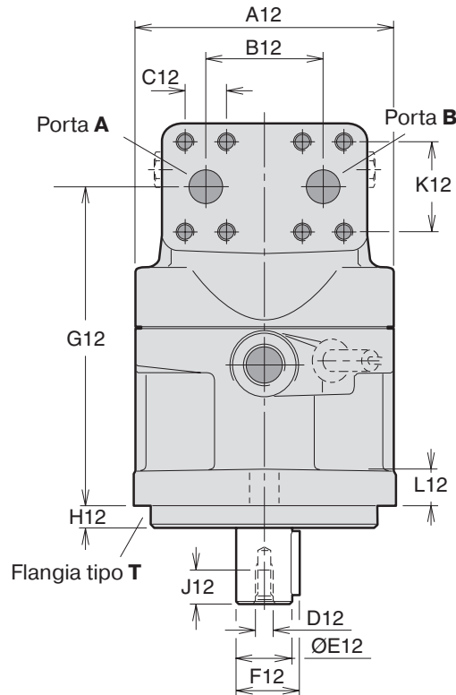
Abb. F10-80 mit 2-Loch Flansch
