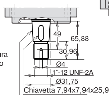
Albero conico con chiavetta "V" SAE J744 32-3 (C)
