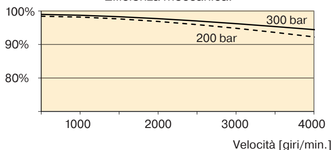
Efficienza meccanica.
