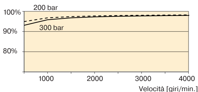
Efficienza volumetrica.
