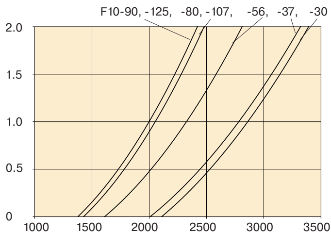
Diagramma 2 Pressione in ingresso min richiesta (F10-A)
