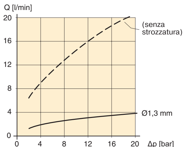
Portata/differenza di pressione (porta A o B al serbatoio).
