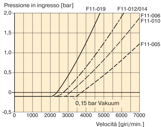
Diagramma 1. Pressione in ingresso min richiesta
