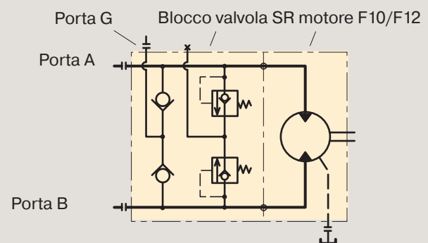
Schema del blocco valvola SR.
