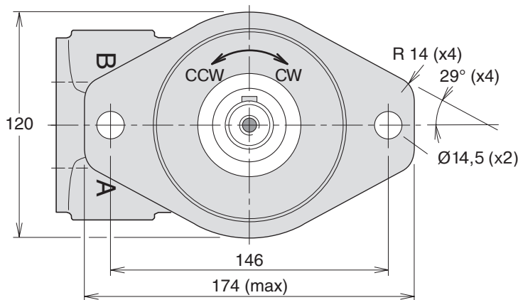
Flangia di montaggio tipo S SAE 'B' ( SAE J744c)
