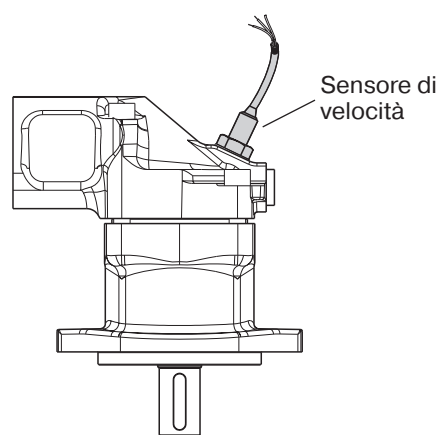
F11-14 con sensore di velocità.
