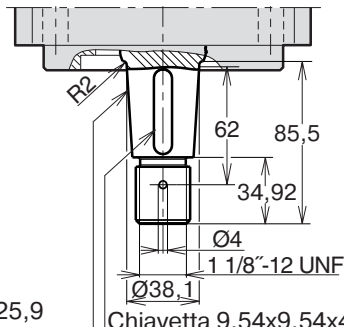
Albero conico con chiavetta "V" SAE J744 38-3 (C-C)
