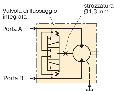
Schema idraulico.
