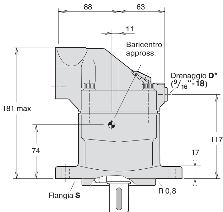
Flangia di montaggio tipo S SAE 'B' (SAE J744c)
