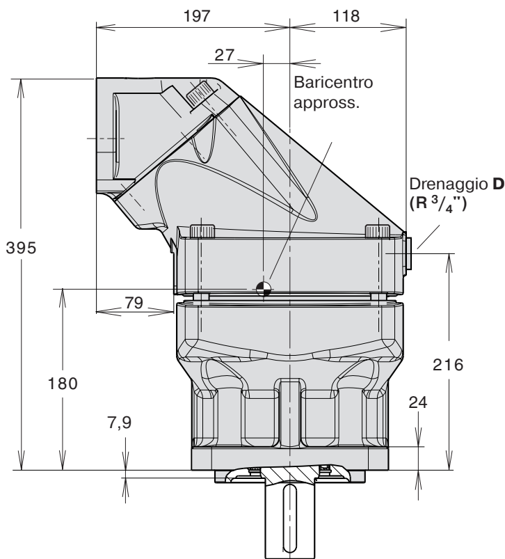
Flangia di montaggio tipo S SAE 'D' (SAE J744c)
