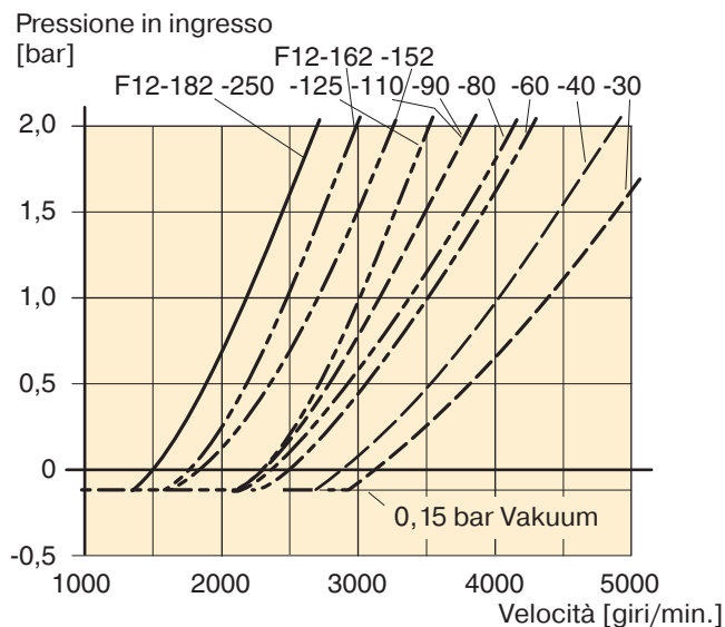
Diagramma 2. Pressione in ingresso min richiesta pompa (F12-L o -R).
