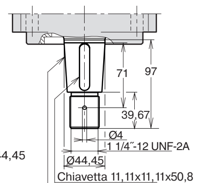
Albero conico con chiavetta "V" SAE J744 44-3 (D&E)
