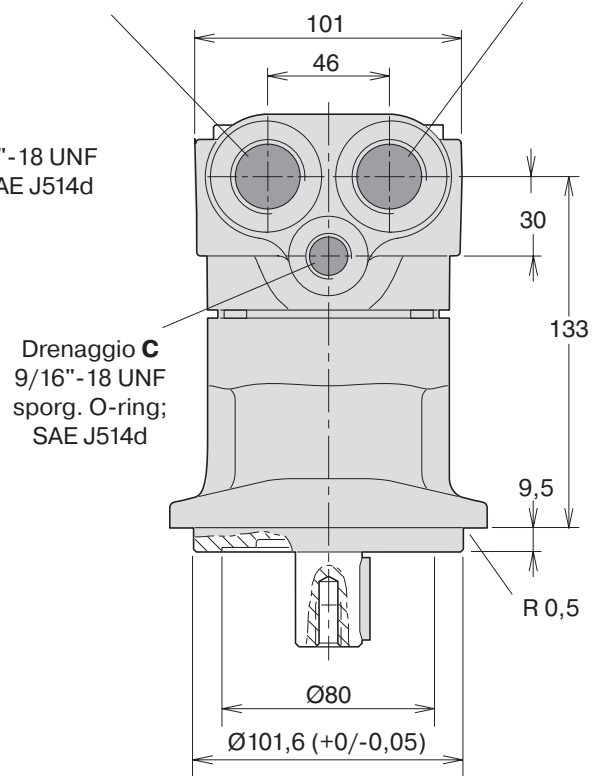
Porta principale A 1 1/16" - 12 UN sporg. O-ring; SAE J514d
