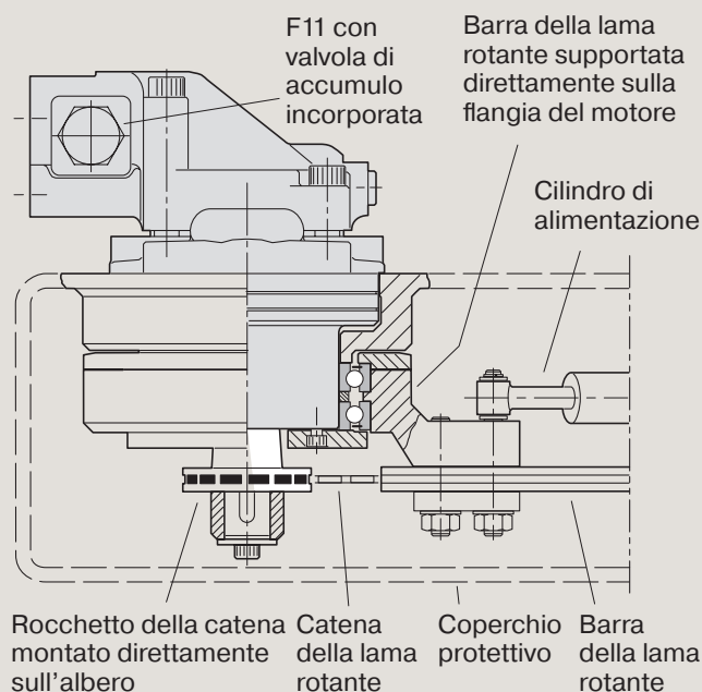
Esempio di installazione della lama rotante catena (F11-10 in figura)
