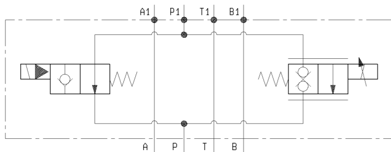
Schema Funzionale
