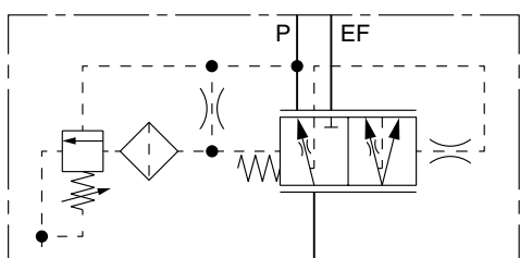
Ripartitore di flusso con priorità con R/V pilotato Funzione "C"
