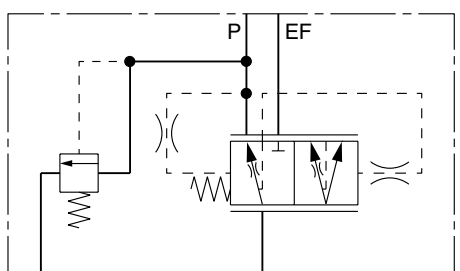
Ripartitore di flusso con priorità con R/V piena portata Funzione "B"
