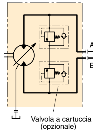
T12 con valvole a cartuccia.
