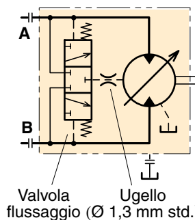
Schema idraulico - V14 con valvola di flussaggio incorporata.
