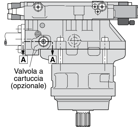
V14- 110 (controllo EP) con valvole di scarico a cartuccia.
