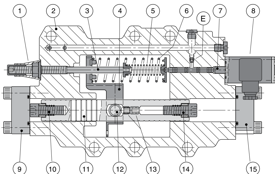
Sezione del modulo di controllo EP.
