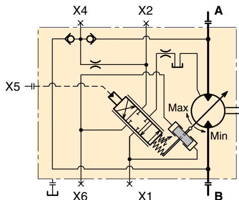
Schema ACE 01 I (bobina in pos. centrale bilanciata).
