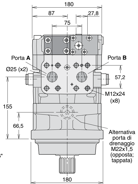
In figura: V14-110-ISO con compensatore AC
