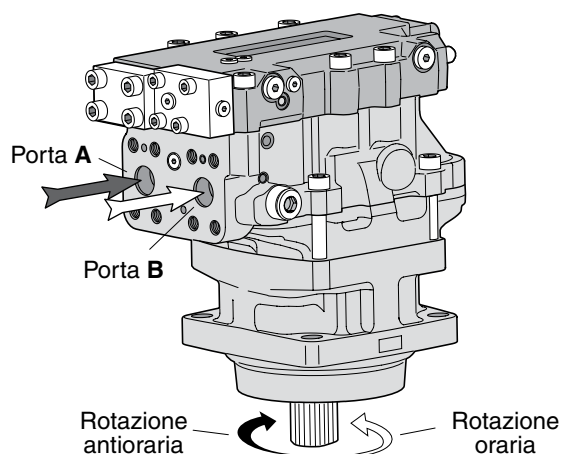
Direzione di rotazione / portata motore V14 (qui con compensatore AC).
