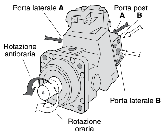
Direzione di rotazione / portata motore V12 (qui con compensatore AC; coperchio terminale in pos. T).
